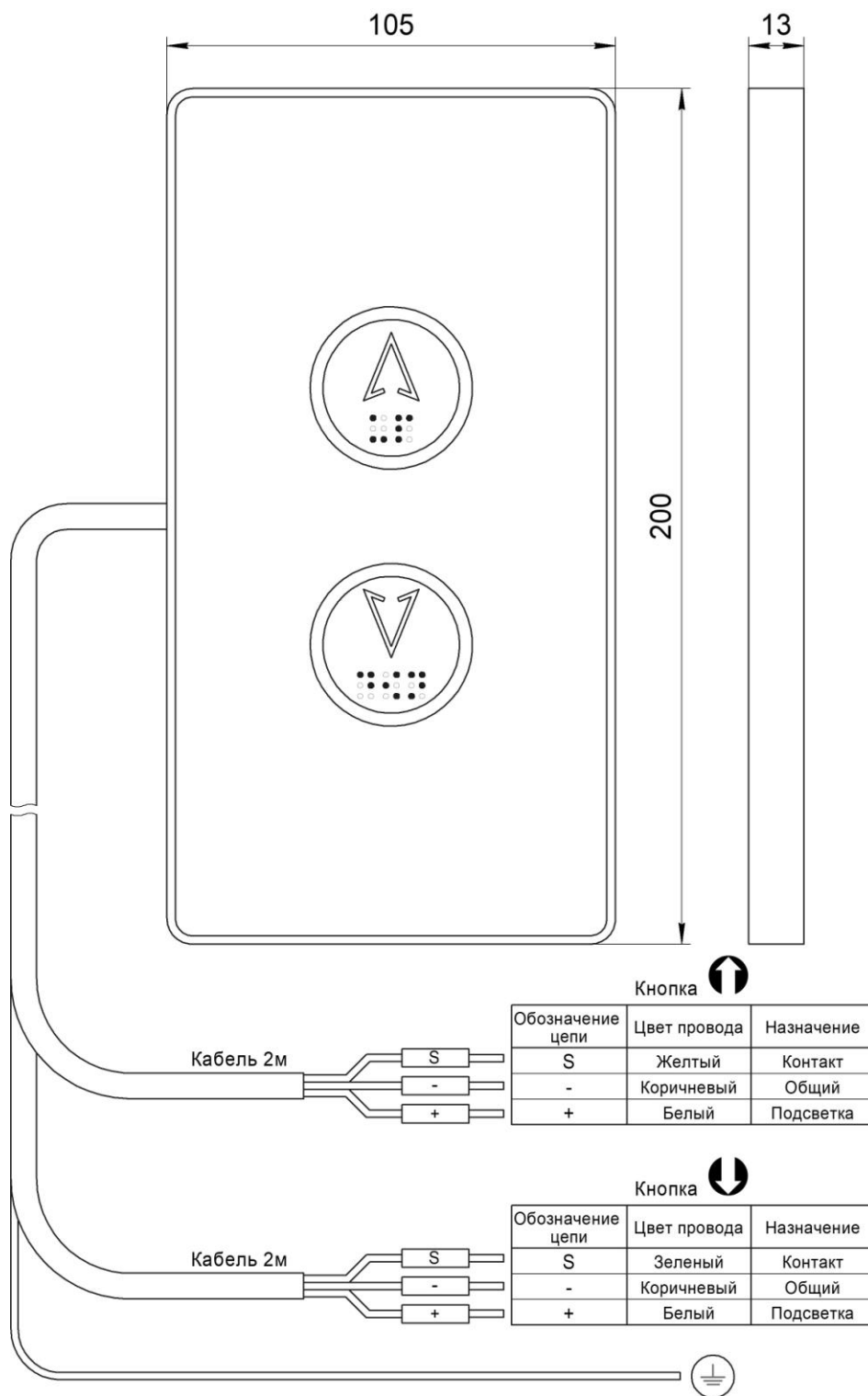
Рис.1 Внешний вид, габаритные и установочные размеры Вызывного поста МАЛАХИТ НШЕК.468381.063-01
